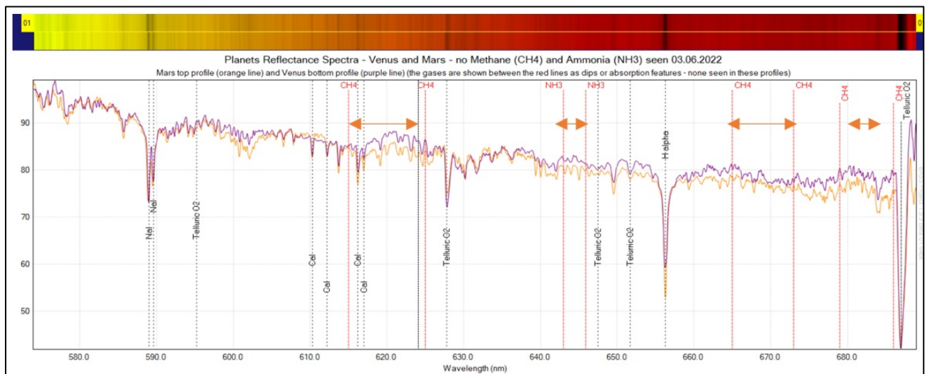
Fig 2. Mars and Venus
