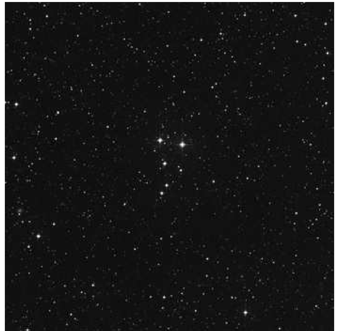
STREICHER 44 – DSH J2123.1-6447 Pavo
