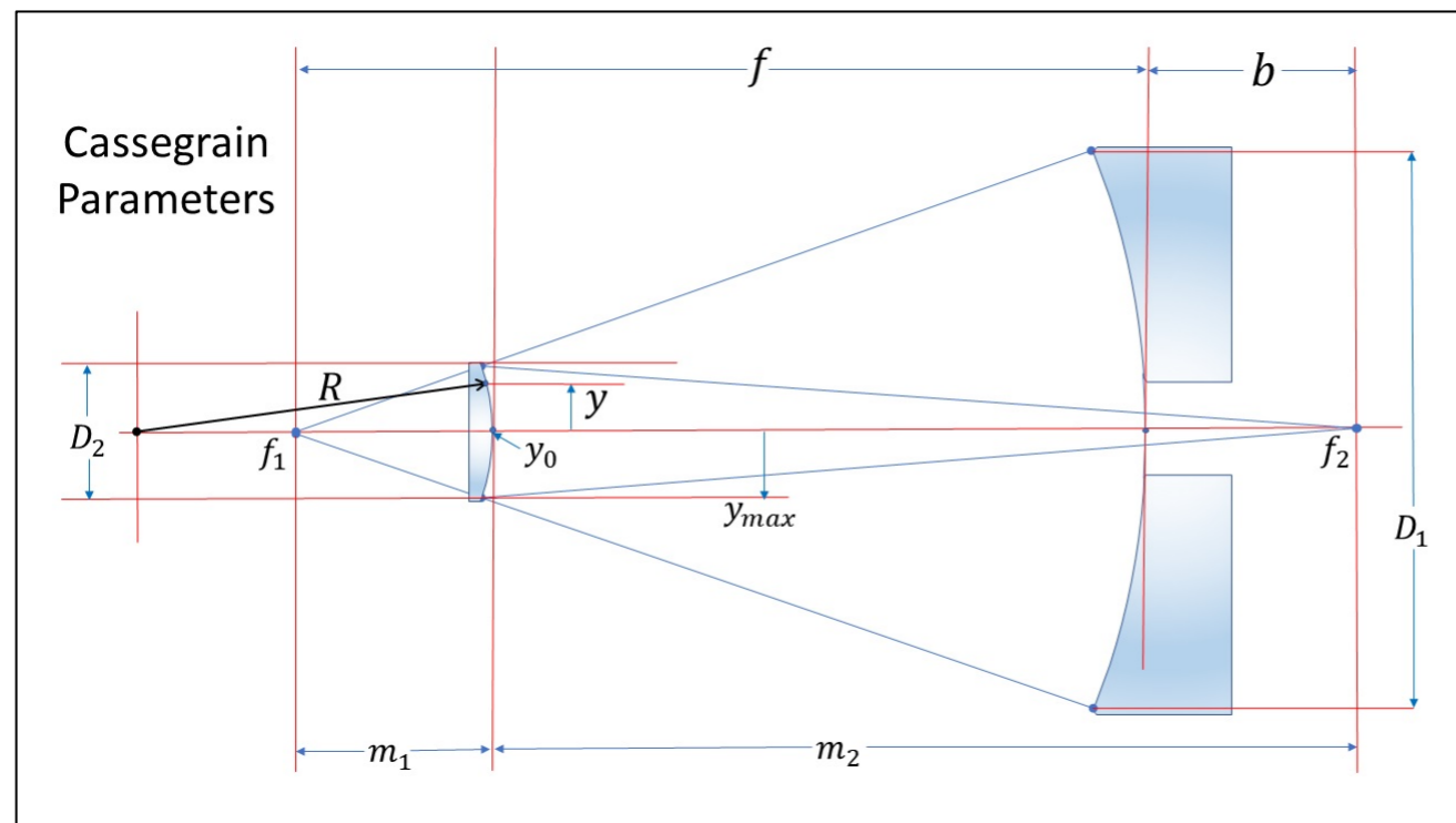
Fig 2. Cassegrain parameters
